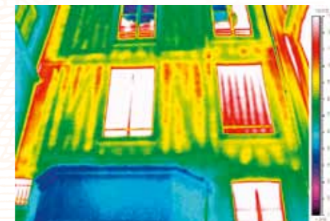
Effet de paroi froide sur un mur en pans de bois et moellons et thermographie infra-rouge de façade.
