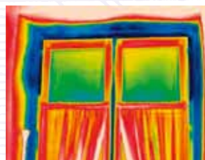
Mise en exergue de la déperdition thermique entre le dormant et l'ouvrant d'une fenêtre ancienne par thermographie infra-rouge (zone en bleue)
